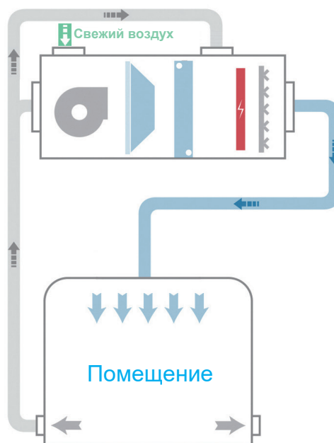
Двухступенчатое всасывание
