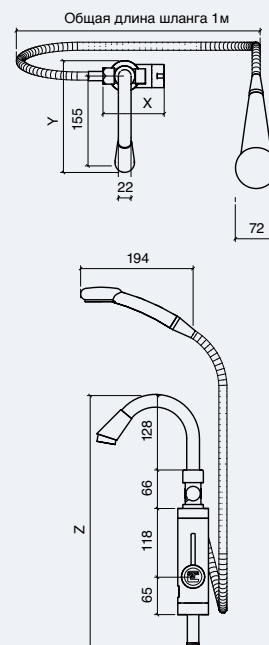
Мелкие отверстия на душевой лейке создают комфортный напор теплой воды для мытья
