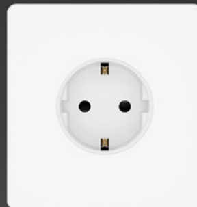
Розетка с заземляющим контактом, защитными шторками, 16А, 250В
