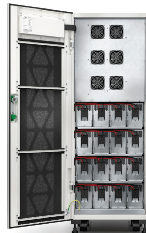
Uniprom UPS 3S, 40 кВА с батареями внутри
