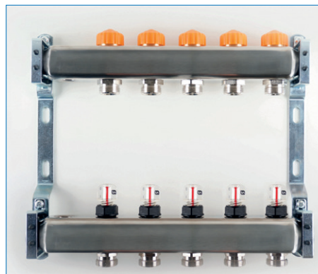
DYNA-if mit autom. Durchflussregelung
