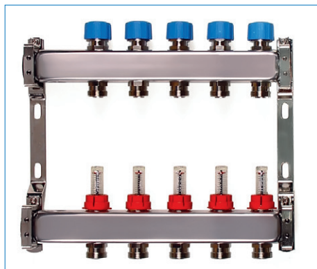
VA-FBif mit Durchflussmengenmesser
