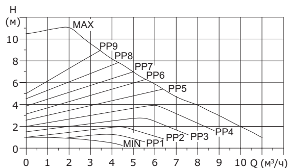
Рис. 42 Кривые режима управления пропорционального изменения давления
