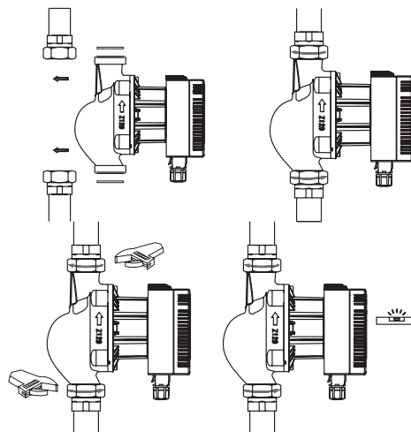
Рис. 39 Монтаж насоса
