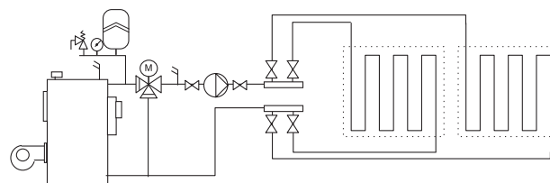
Рис. 27 Система «тёплых полов»
