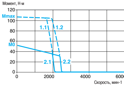
1.1 Пиковый момент, 3-фазная сеть 400 В 1.2 Пиковый момент, 3-фазная сеть 480 В 2.1 Длительный момент, 3-фазная сеть 400 В 2.2 Длительный момент, 3-фазная сеть 480 В
