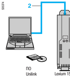
Соединение ПК и сервопреобразователя Lexium 15
