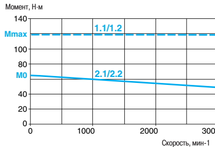
С сервопреобразователем LXM 15HC11N4X 400/480 В, 3-фазная сеть
