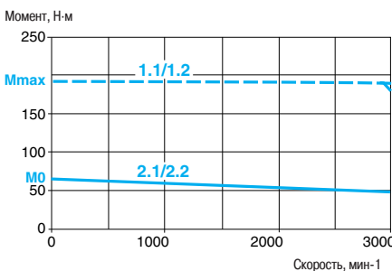
С сервопреобразователем LXM 15HC20N4X 400/480 В, 3-фазная сеть
