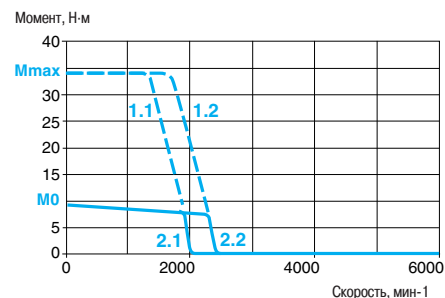
С сервопреобразователем LXM 15MD40N4 400/480 В, 3-фазная сеть
