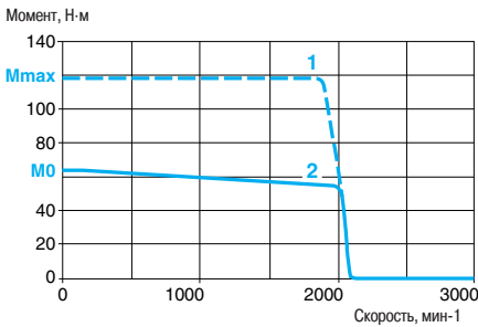
С сервопреобразователем LXM 15HC20N4X 400/480 В, 3-фазная сеть
