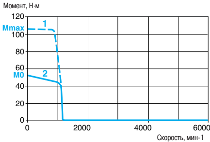
1 Пиковый момент 2 Длительный момент
