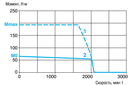
С сервопреобразователем LXM 15HC20N4X 230 В, 3-фазная сеть
