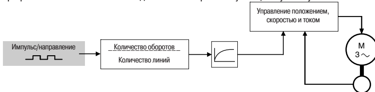
Режим “электронный редуктор”
