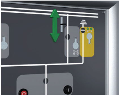
Переключатель шибровой заслонки отверстия для рукоятки управления разъединителем и заземлителем
