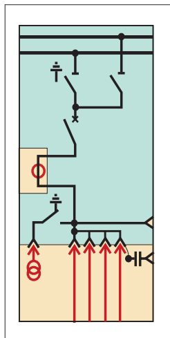
Ячейка с силовым выключателем
