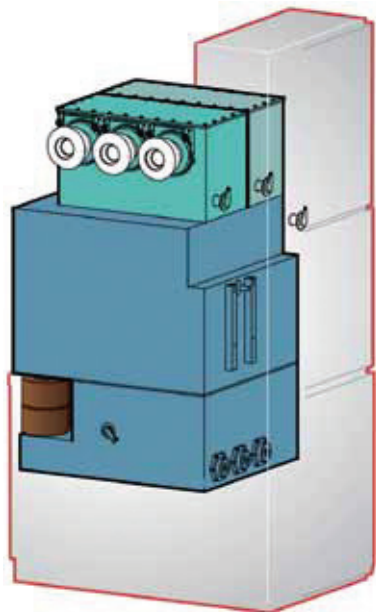
Ячейка секционирования (SBB), I_r \leq 2000 A
