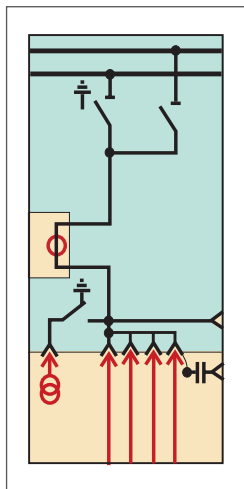
Ячейка с разъединителем / заземлителем
