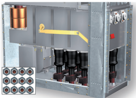
Кабельный ввод с внутренним конусом до 35 кВ, 4 подключения на фазу, размер 2 (800 А) или размер 3 (1250 А) с ТН на вводе
