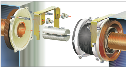
Компоненты B-Link
