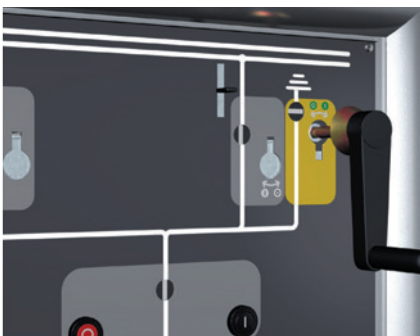
Управление заземлителем (ВКЛ - ОТКЛ)
