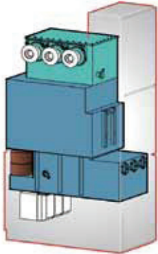
Ячейка ввода / отходящей линии Кабельные адаптеры с внутренним конусом
