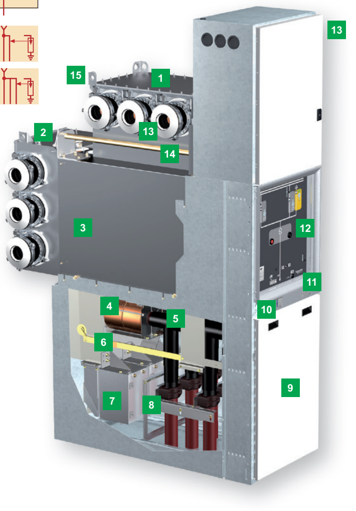
Ячейка ввода / отходящей линии (DBB)
