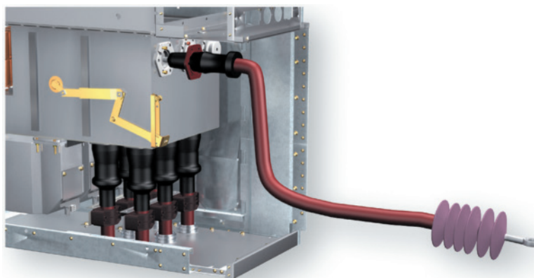
Испытательный кабель для КРУЭ с внутренним конусом
