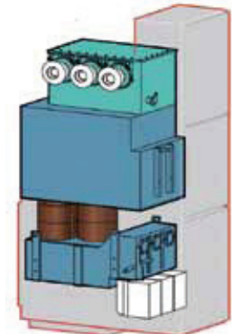
Ячейка овода / отходящей линии Кабельные адаптеры с внутренним конусом внутри кабельного отсека
