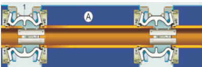
Компоненты B-Link
