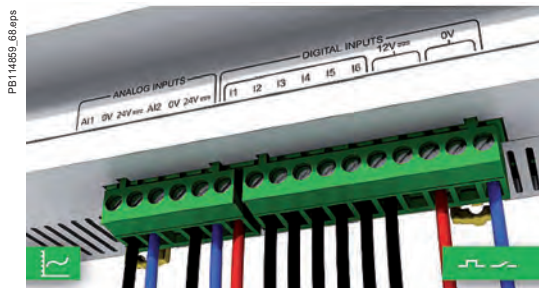
Питание аналоговых и дискретных входов
