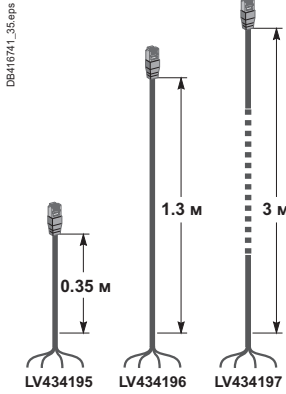
Кабель ULP cord выключателя
