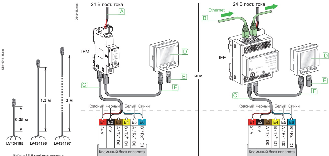
Кабель ULP cord выключателя
