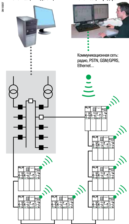
Автоматизация подстанции
