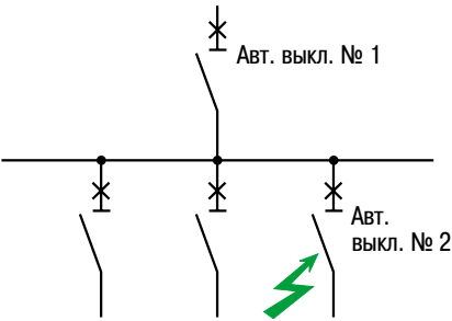
Селективность между автоматическими выключателями распределительной сети
