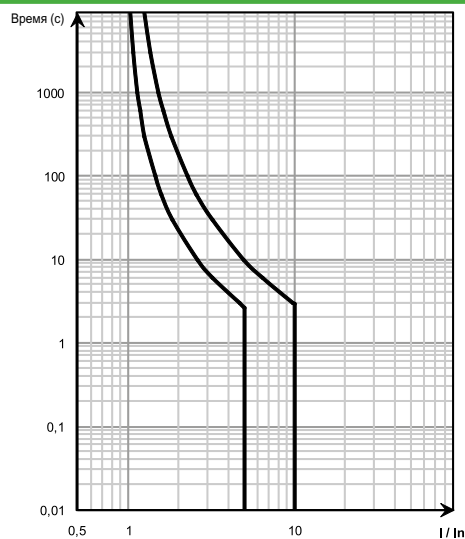
Кривая С
