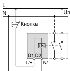
Расцепители iMN / iMNs с питанием от главной сети
