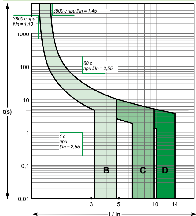
Кривые B, C, D до 4 А
