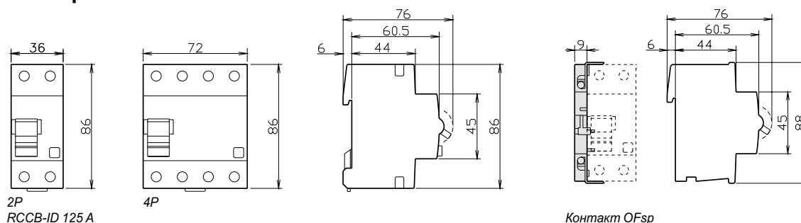
Контакт OFsp
