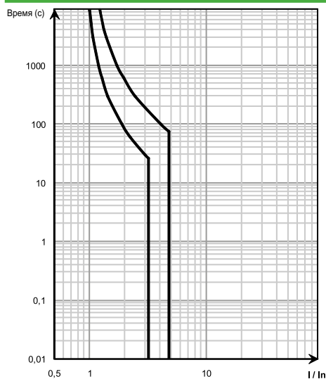
Кривая В
