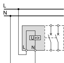
Контроль однофазной системы питания
