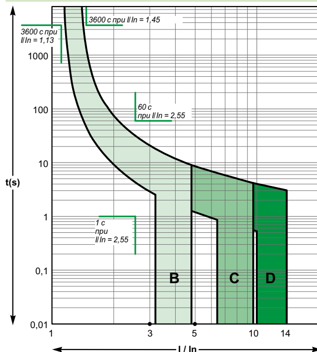
Кривые B, C, D
