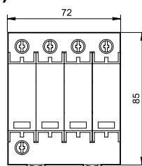
3P+N, 4P
