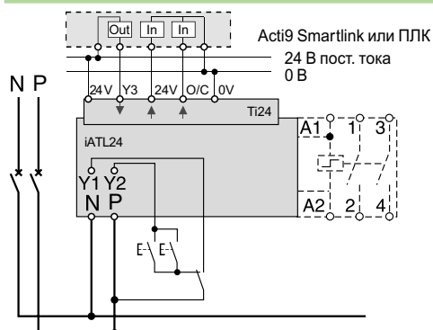
Разводка с выделенным переключателем управления 230 В пер. тока и 24 В пост. тока
