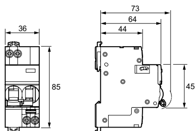
АВДТ 1P+N
