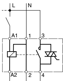
Фальш-модуль, № по каталогу A9A27062
