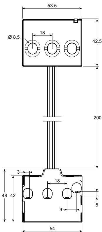
3P+N
