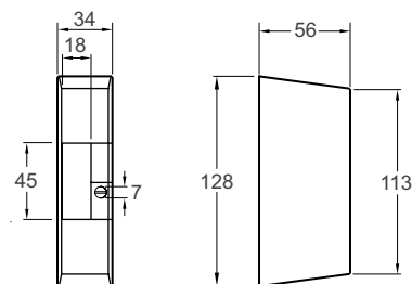
Крепление для настенного монтажа
