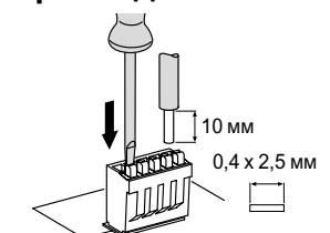
Разъем, № по каталогу A9XC2412
