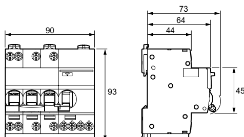
АВДТ 3P+N
