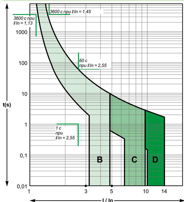
Кривые B, C, D
