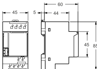
Термостаты ТН4 и ТН7
