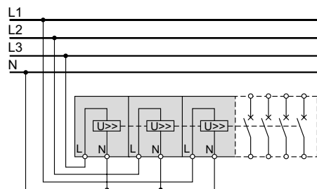
Контроль трёхфазной системы питания
