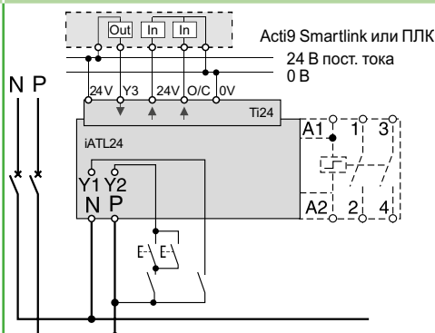
Разводка без выделенного переключателя управления 230 В пер. тока и 24 В пост. тока
