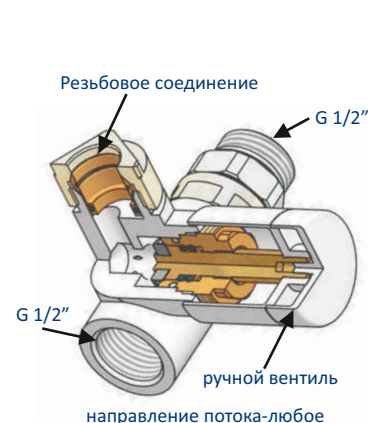
Клапан с ручным вентилям
