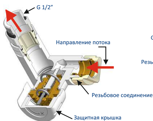
Клапан термостатический
