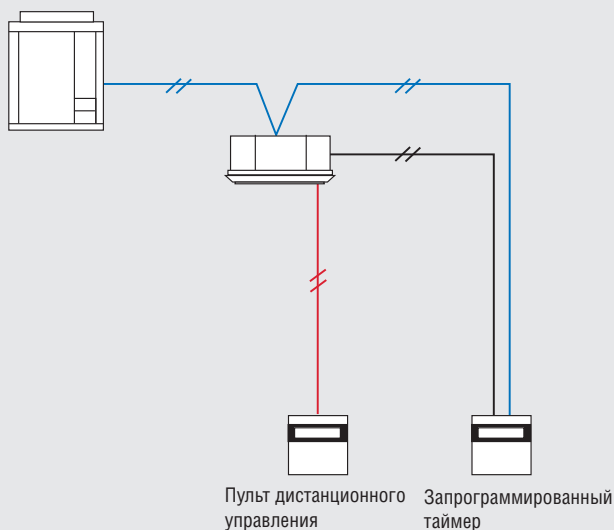
Пример соединения 1 (Питание от кондиционера в помещении)
