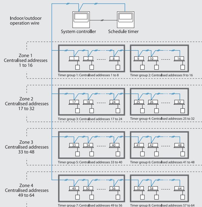
Пример соединения 2 (Питание от центрального пульта управления)
