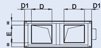
CFR 110 ÷ 410 CFR-PHE 110 ÷ 410
