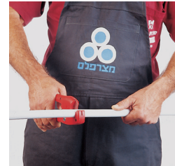
1 Резка трубы
