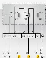
Монтажные схемы Для крышных вентиляторов
