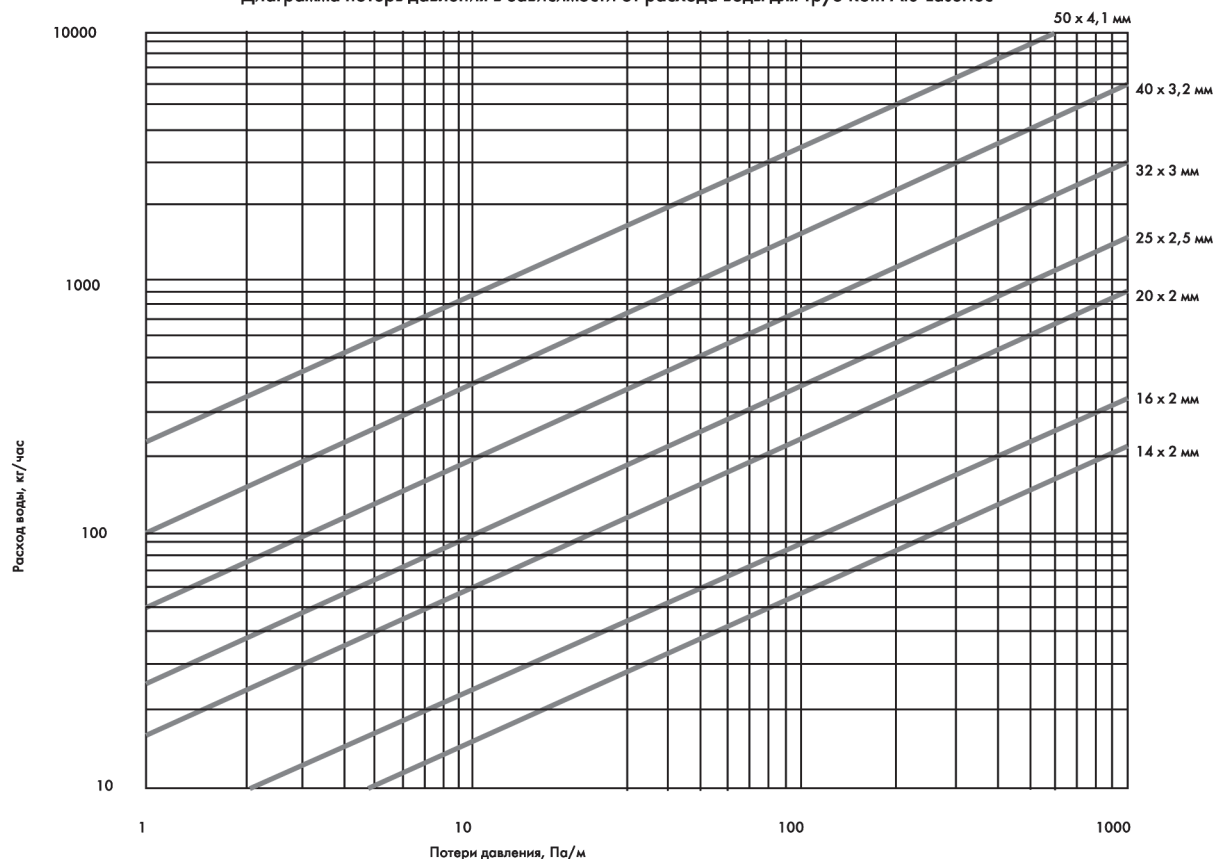
Диаграмма потерь давления в зависимости от расхода воды для труб Roth Alu-Lasertec
