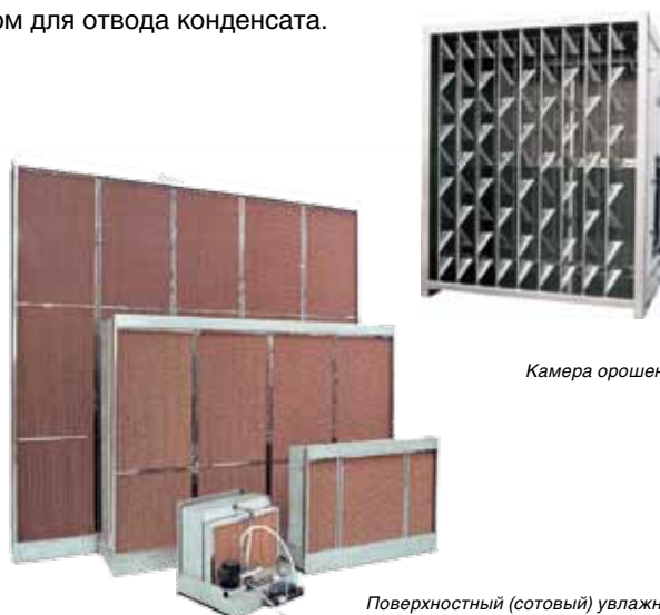
Поверхностный (сотовый) увлажнитель
