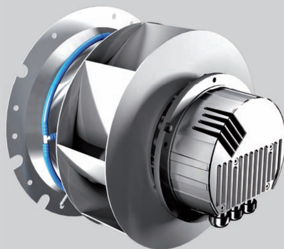
Колесо свободного вращения для применения в качестве приточного вентилятора в ж/д установках климатизации пассажирских купе.
