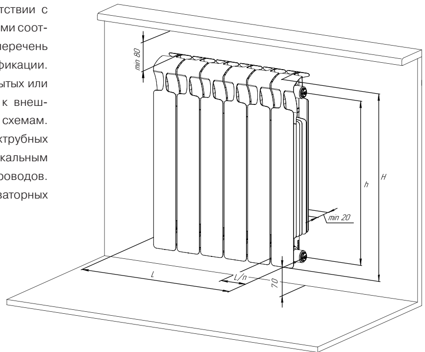
Рис 1. Схема настенного монтажа радиатора
