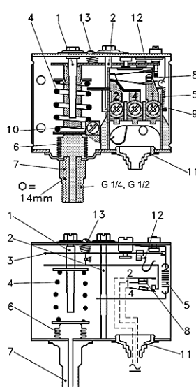
Рис. 1. Устройство реле давления КРІ
