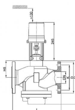
Клапан AQF-R DN 65 с приводом
