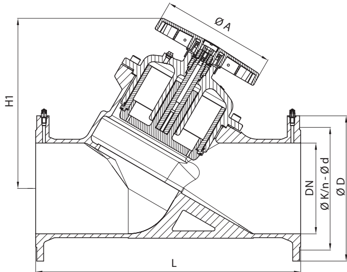
Клапан MNF-R2 DN200–400
