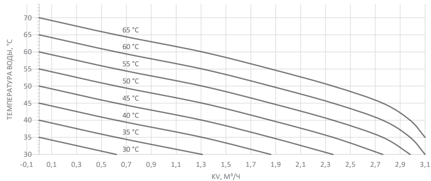
Зависимость Kv клапана АНТ-R DN25 от его настройки и температуры воды
