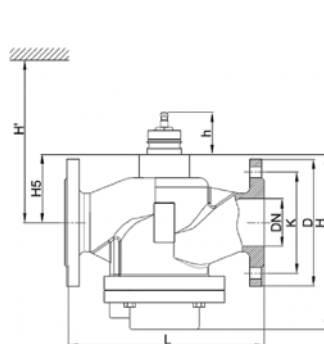
Клапан AQF-R DN 65-200
