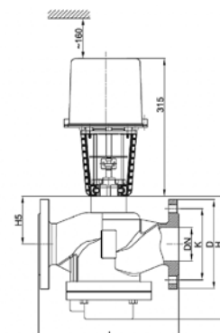
Клапан AQF-R DN 80-200 с приводом
