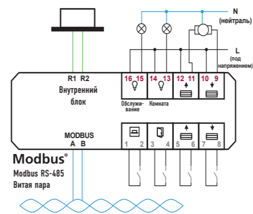
Пример входа / выхода: конфигурация проводки для Варианта 2
