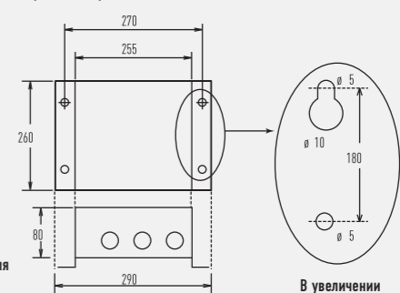
Контроллер входа/выхода Seri-Para I/O для внешнего блока (CZ-CAPDC2)
