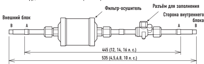
Комплект оборудования VRF Renewal Kit (CZ-SLK2)
