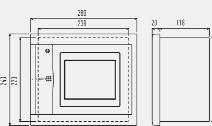
Интеллектуальный контроллер (CZ-256ESMC2)
