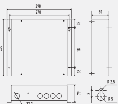
Адаптер связи (CZ-CFUNC2)
