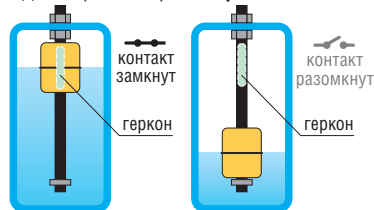
ПДУ с нормально-разомкнутым контактом
