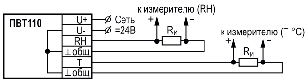
Схема подключения ПВТ110-А (тип выходного сигнала-0-10 В)
