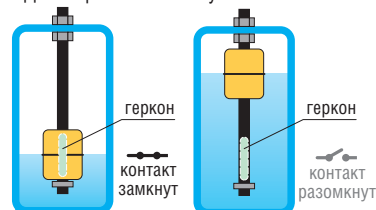
ПДУ с нормально-замкнутым контактом
