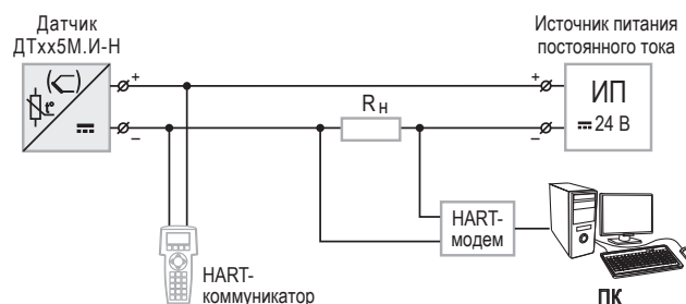
Схема передачи цифрового сигнала от датчика к устройству, поддерживающим HART-протокол
