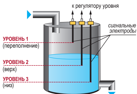
Металлический резервуар, вертикальный монтаж
