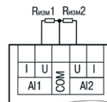
Подключение резистивных датчиков
