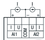
Подключение датчиков с токовым выходом
