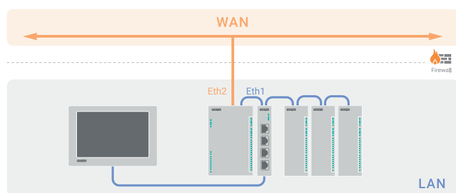
Схема 1. Порт Ethernet 1 подключен к локальной сети (LAN). Порт Ethernet 2 используется как отдельный изолированный сетевой интерфейс для подключения к глобальной сети (WAN), защищенный межсетевым экраном.
