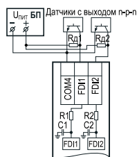
Подключение к входам типа «ДС» датчиков с выходом п-п-п
