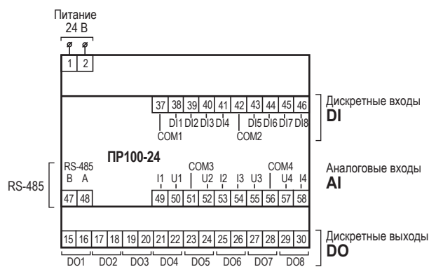
Схема расположения и назначение клемм ПР100-24
