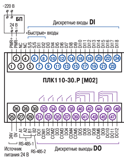
Схема расположения и назначения клемм ПЛК110-24.30.Р [M02]
