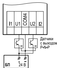
Схема подключения к универсальным входам, работающим в дискретном режиме трехпроводных дискретных датчиков, имеющих выходной транзистор р-п-р-типа с открытым коллектором
