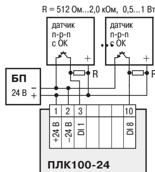
ПЛК100-24, датчик п-р-п-типа
