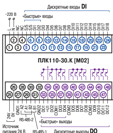
Схема расположения и назначения клемм ПЛК110-220.30.К [M02]
