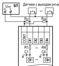
Подключение к входам типа «Д» датчиков с выходом р-п-р
