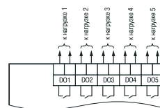
Схема подключения нагрузки к ВЭ типа Р
