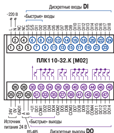
Схема расположения и назначения клемм ПЛК110-220.32.К [M02]
