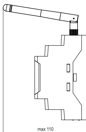
Габаритные размеры Пх210 с антенной
