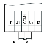
Подключение резистивных датчиков
