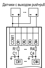
Подключение к входам типа «Д» датчиков с выходом push-pull
