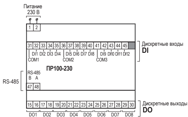
Схема расположения и назначение клемм ПР100-230
