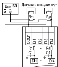
Подключение к входам типа «Д» датчиков с выходом п-р-п
