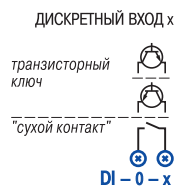
Схема подключения дискретных входов ПЛК100
