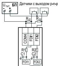
Подключение к входам типа «ДС» датчиков с выходом р-п-р
