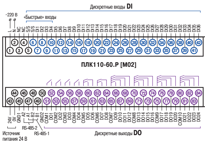
Схема расположения и назначение клемм ПЛК110-220.60.Р [M02]
