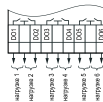
Схема подключения ВЭ типа «Р»
