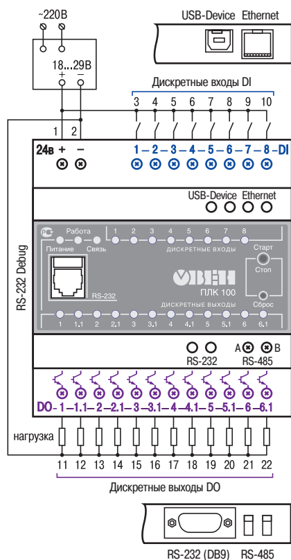
Схема подключения ПЛК100-24.К
