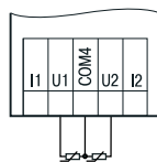
Подключение ТС к аналоговому входу
