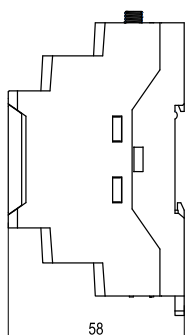
Габаритные размеры Пх210 без антенны
