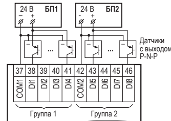
Подключение трехпроводных дискретных датчиков, имеющих выходной транзистор p-n-p-типа с открытым коллектором (для модификаций ПР100-24)
