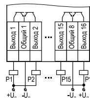
Подключение нагрузки к выходу типа КТ
