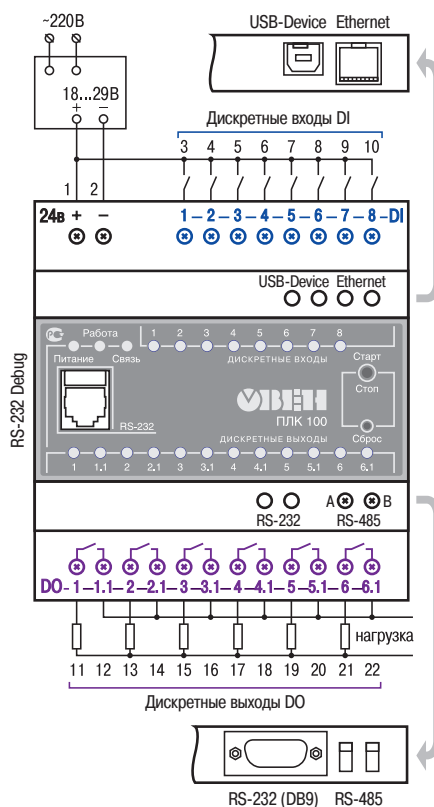
Схема подключения ПЛК100-24.Р
