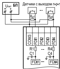
Подключение к входам типа «ДС» датчиков с выходом п-р-п
