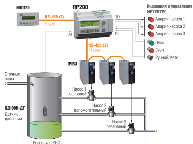
Автоматизация КНС
