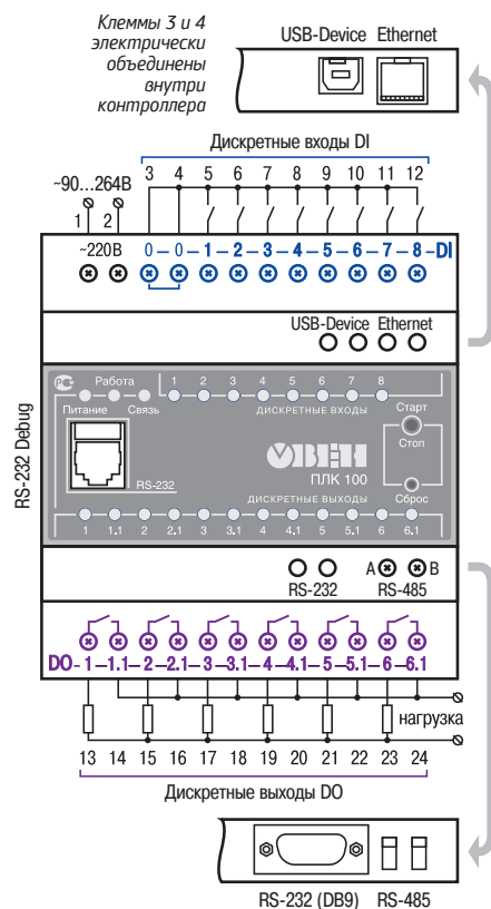
Схема подключения ПЛК100-220.Р
