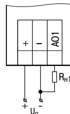
Схема подключения к аналоговому выходу токовой нагрузки
