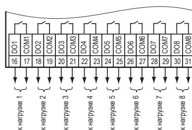
Подключение нагрузки к выходным элементам (ВЭ) типа Р (электромagnetное реле)
