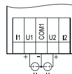
Подключение датчиков с выходом в виде напряжения
