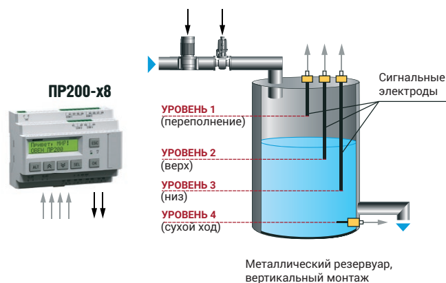
Сигнализатор уровня
