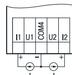
Подключение датчиков с выходом в виде тока
