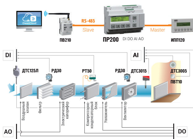
Управление вентиляцией
