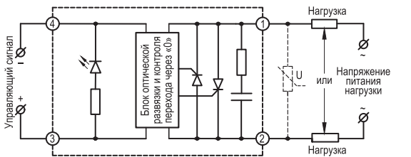
Схема включения ТТР серии HDH-xx44.ZD3 (выход – SCR-тиристор)
