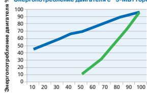
Относительная мощность горелки в %
