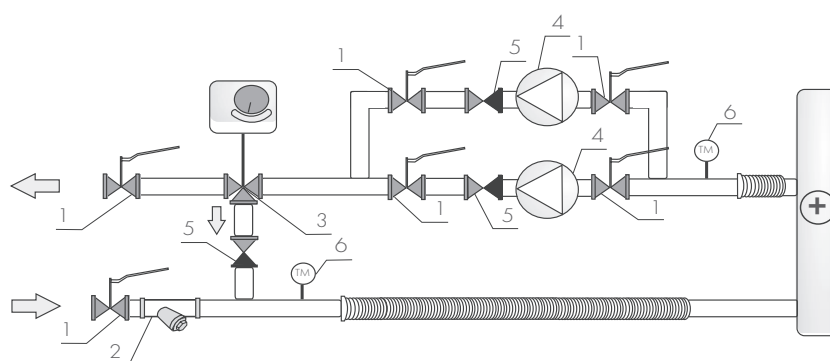
Решение с резервным насосом для ПВУ и канального оборудования
