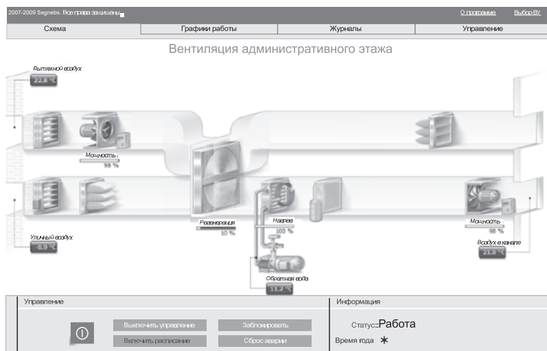
Рисунок 1 – Отображение технологической схемы
