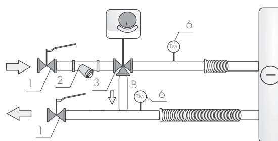
Решение с прямым принципом сборки для ПВУ и канального оборудования
