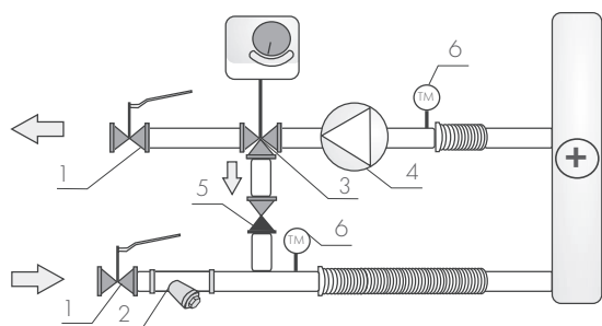
Стандартное решение для ПВУ и канального оборудования
