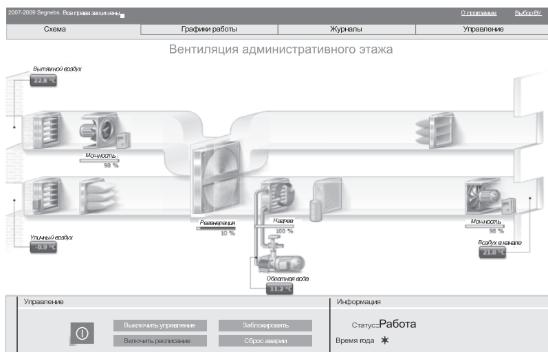
Рис.1 Отображение технологической схемы
