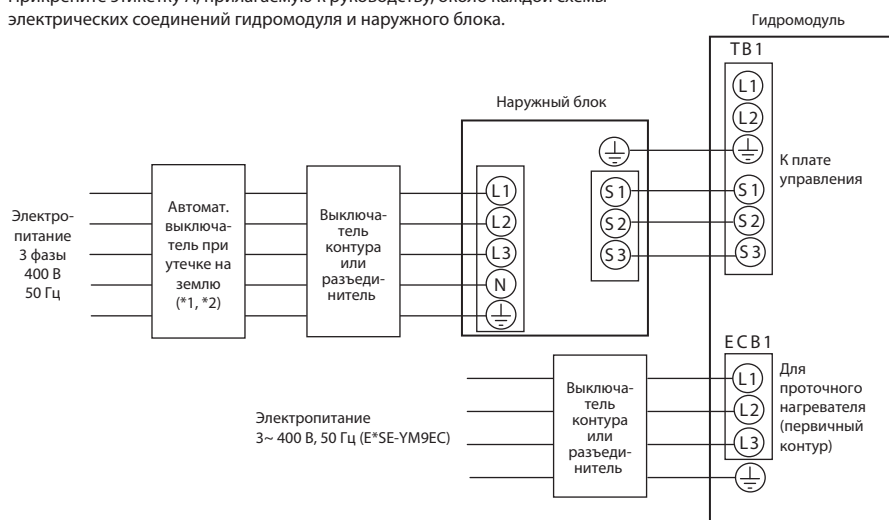
Рис. 3.2.15 Электрические соединения, 3 фазы
