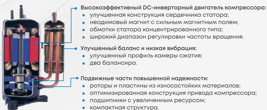
Двухроторный инверторный компрессор
