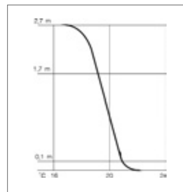
Рис. 3. Распределение температуры в помещении с подпольным отоплением.
