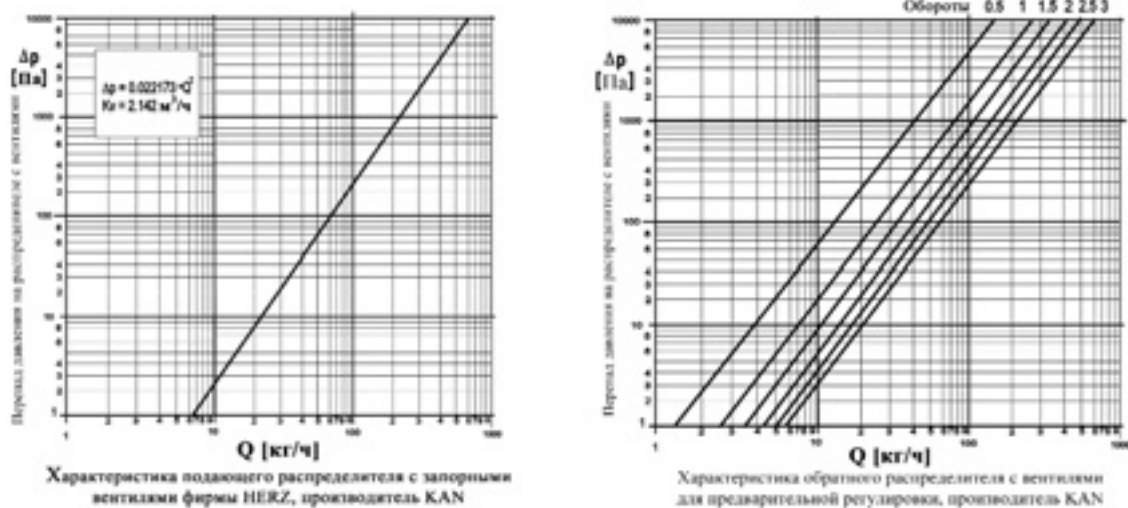
Рис. 41. Характеристика вентилей, встроенных в распределитель.
