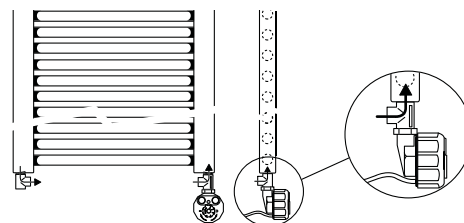
Подсоединение смешанного типа.
