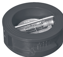
КЛАПАН ОБРАТНЫЙ МЕЖФЛАНЦ. СТВОРЧАТЫЙ NRD-W
