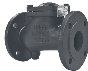
КЛАПАН ОБРАТНЫЙ ШАРОВЫЙ ФЛАНЦЕВЫЙ NRB-F
