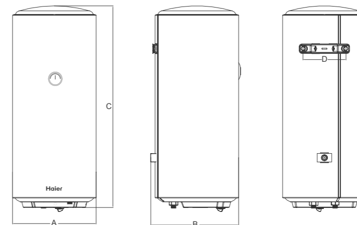
Вид спереди
