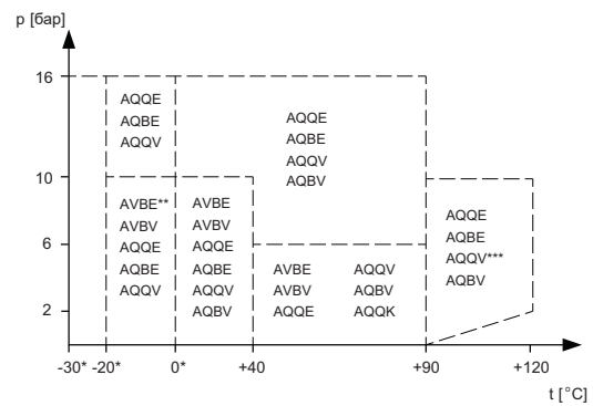
Рис. 13 График выбора уплотнения вала
