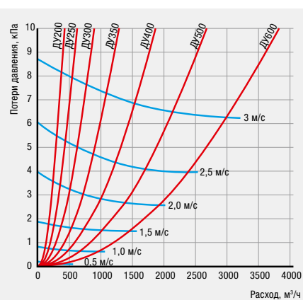
Стальные от Ду 200 до Ду 500
