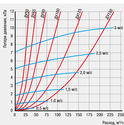
Стальные от Ду 50 до Ду 150
