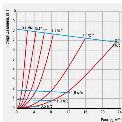
Полимерно-композитные от 22 мм до 2"
