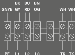
Схема 2 (400 В, 3 ф, 50 Гц.)
