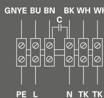
Схема 1 (230 В, 1 ф, 50 Гц.)
