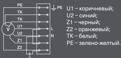
Схема 2 (230 В, 1 ф.)
