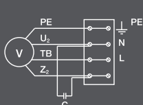
Схема 1 (230 В, 1 ф.)
