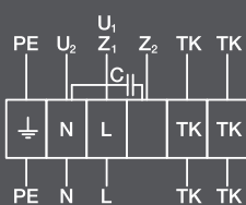
Схема 1 (230 В, 1 ф.)
