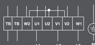
Схема 2 Δ — 400 В, 3 ф.
