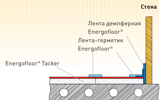
Схема установки тёплого пола
