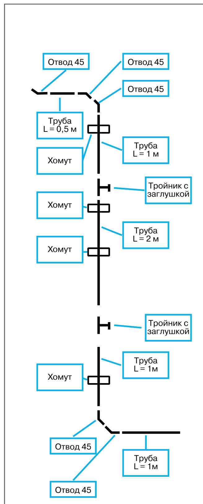
Вертикальный участок
