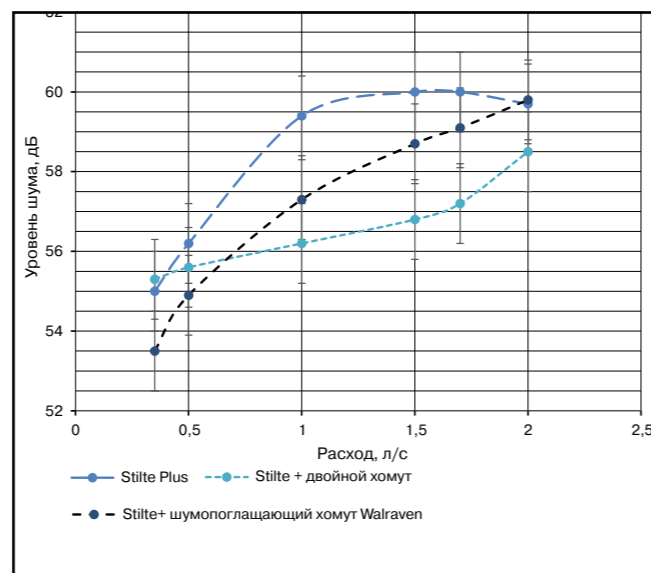
Горизонтальный участок
