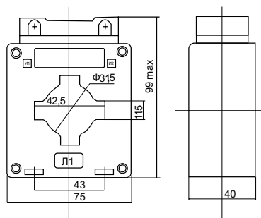
ТШП-0,66-40
