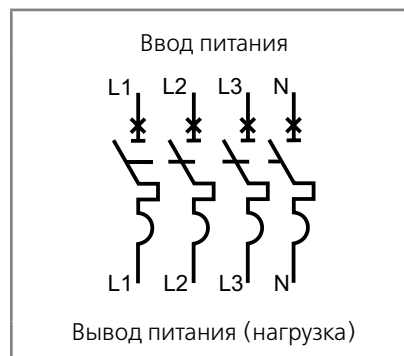
ВА-338Е 4P
