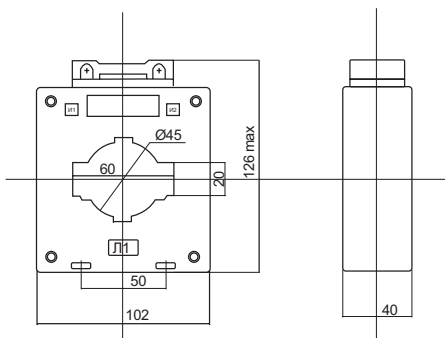
ТШП-0,66-60
