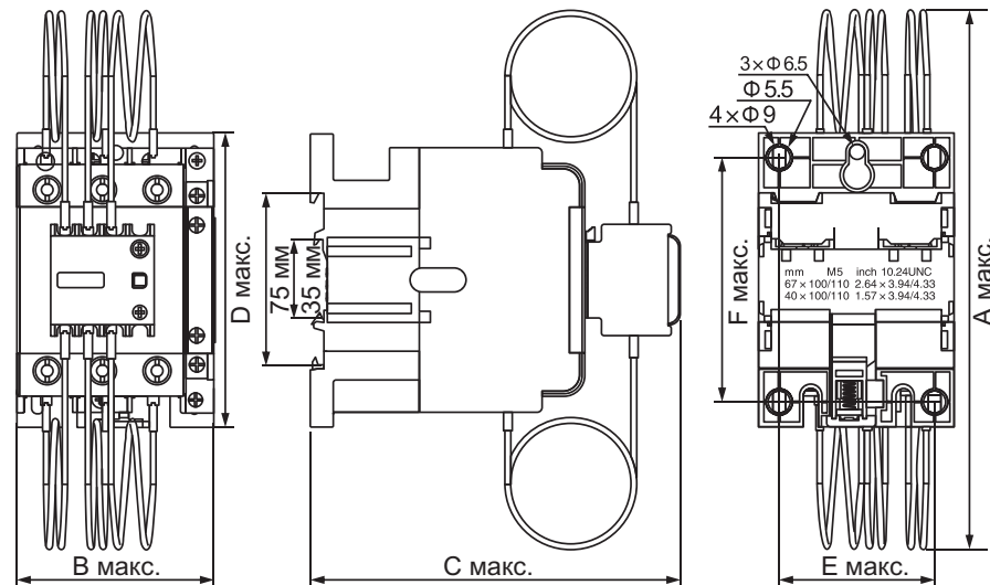
KM-102-CAP 30 ~ 60 кВАр
