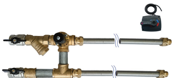
Узел регулирования воздухоохладителя
