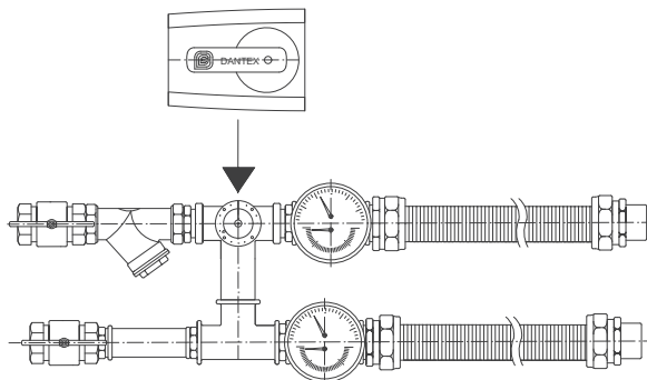
Узел регулирования воздухоохладителя с термоманометрами
