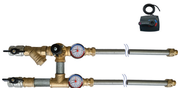
Узел регулирования воздухоохладителя с термоманометрами
