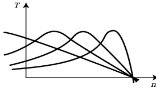
Рис. 1.20 Характеристики крутящего момента при изменении сопротивления ротора
