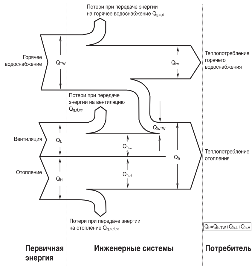
Рис. 6. Энергетический баланс отопления, вентиляции и горячего водоснабжения здания: Q_{TW} , Q_L и Q_H – годовые затраты теплоты соответственно на горячее водоснабжение, вентиляцию и отопление; Q_{tw} – годовая потребность теплоты на горячее водоснабжение; Q_h – годовая потребность теплоты на отопление; Q_{h,TW} , Q_{h,L} и Q_{h,H} – доля в годовой потребности теплоты на отопление теплопоступлений соответственно от систем горячего водоснабжения, вентиляции и отопления; Q_{g,s,d,ce} – годовые энергопотери соответственно индексам на производство, аккумуляцию, распределение и передачу теплоты
