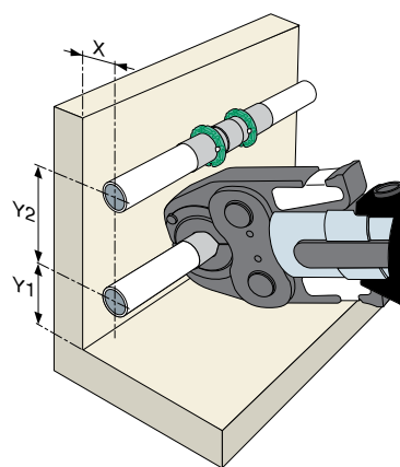
рис.2: Монтаж у основания стены
