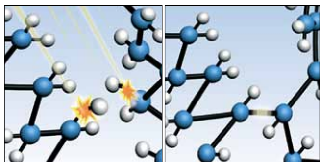
Физическая сшивка (облучение трубы HDPE высокой энергией, например электронно-лучевой или гамма-излучением)
