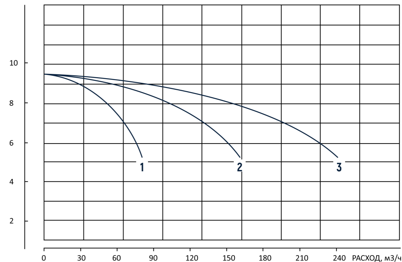
НАПОР, М PFFS NES 80-65-165-2,2/4
