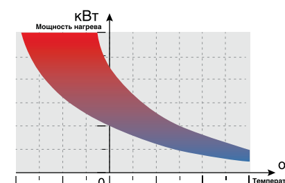
Металлокерамические нагревательные элементы Ballu имеют свойство автоматической терморегуляции. Чем выше их температура, тем больше электрическое сопротивление, меньше потребляемая мощность и меньше нагрев. Это исключает перегрев и обеспечивает высокую экономичность расхода электроэнергии
