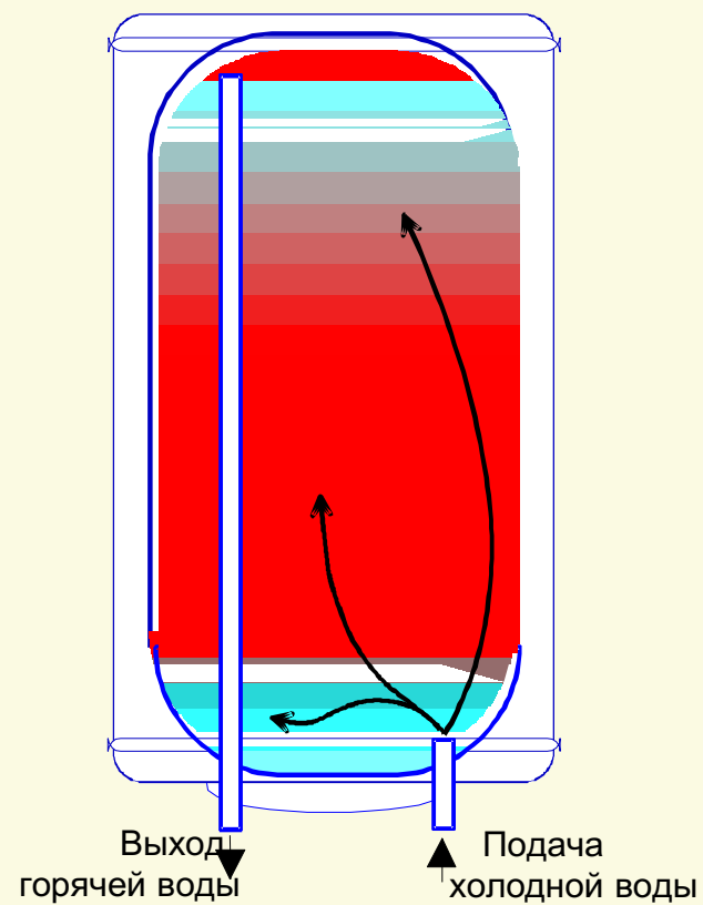
Стандартный водонагреватель
