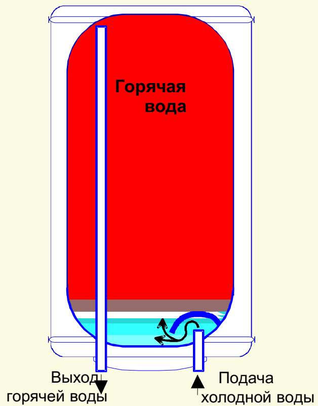
Водонагреватель ATLANTIC
